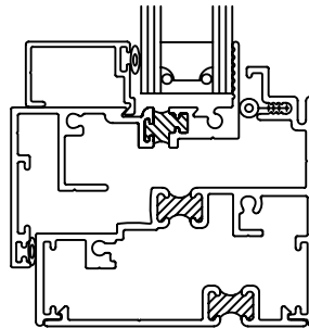
SILL W/O FIN
