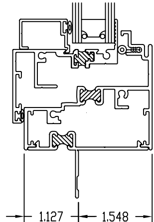
SILL W/REVERSE FIN
